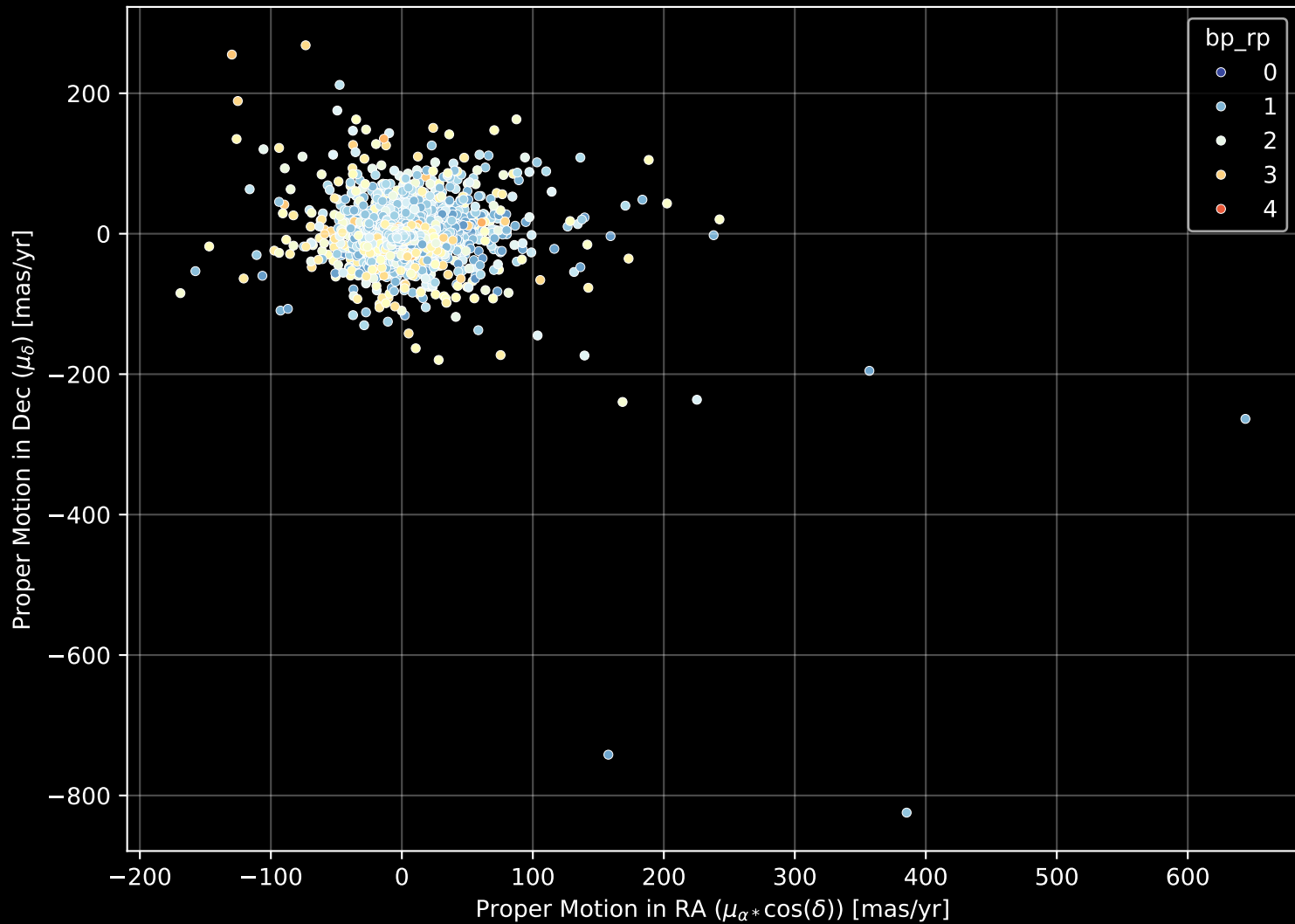
GALAH DR4 Field: [-1] Proper Motion Diagram (n= 7543)
