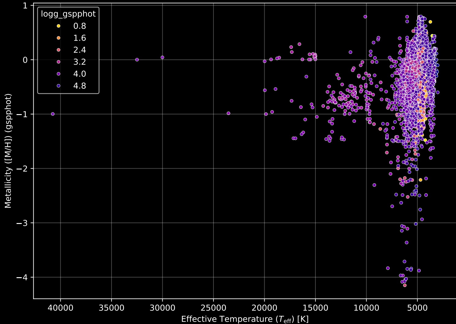
GALAH DR4 Field: [-1] Stellar Population Parameters (n= 7543)
