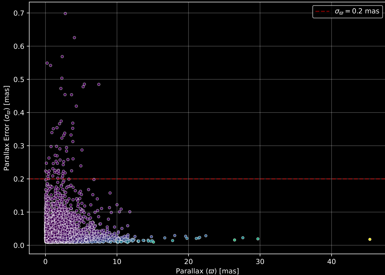
GALAH DR4 Field: [-1] Parallax Quality (n= 7543)
