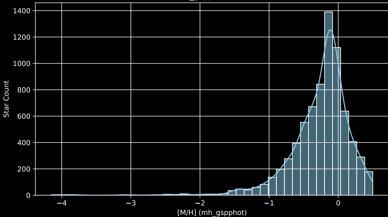
GALAH DR4 Field: [-1] [M/H] (mh_gspphot) (n= 7445)
